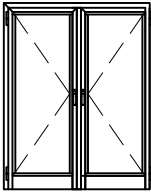
ÇİFT KANAT DIŞA AÇILIR KAPI DOUBLE OUTWARD OPENING DOOR
