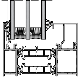
CAM KALINLIĞINA GÖRE CAM ÇITASI SEÇİM TABLOSU KASA-ORTA KAYIT PROFİLİ İÇİN Glazing Bead Selection Table according to the Glass Thickness FRAME-TRANSOM/MULLION profiles.
