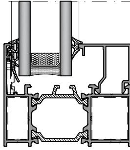
CAM KALINLIĞINA GÖRE CAM ÇİTASI SEÇİM TABLOSU KASA-ORTA KAYIT PROFİLİ İÇİN Glazing Bead Selection Table according to the Glass Thickness FRAME-TRANSOM/MULLION profiles.
