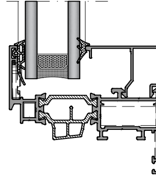
CAM KALINLIĞINA GÖRE CAM ÇİTASI SEÇİM TABLOSU KANAT-KANAT İÇİ ORTAKAYIT-ETEK PROFİLİ Glazing Bead Selection Table according to the Glass Thickness SASH-SASH MULLION-BOTTOM RAIL PRO.
