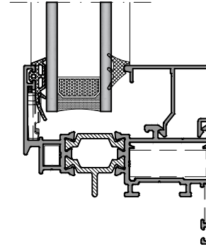
CAM KALINLIĞINA GÖRE CAM ÇİTASI SEÇİM TABLOSU KANAT-KANAT İÇİ ORTAKAYIT-ETEK PROFİLİ Glazing Bead Selection Table according to the Glass Thickness SASH-SASH MULLION-BOTTOM RAIL PRO.
