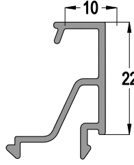
CAM KALINLIĞINA GÖRE CAM ÇİTASI SEÇİM TABLOSU Glazing Bead Selection Table according to the Glass Thickness (LS70-11)
