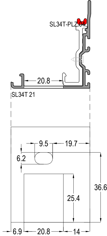
KENET KAPAĞI BOŞLUĞU AÇMA Drill for Interlock Profile Cap SL38T-KP
