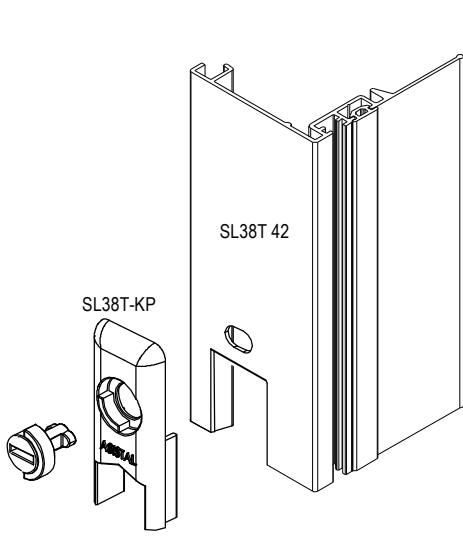
KENET KAPAĞI BOŞLUĞU AÇMA Drill for Interlock Profile Cap SL38T-KP
